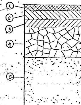
КОНСТРУКЦИИ ТИПА Б-3
