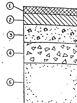
КОНСТРУКЦИИ ТИПА А-1
