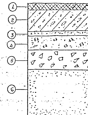
КОНСТРУКЦИИ ТИПА АТ-2 (экспериментальные)
