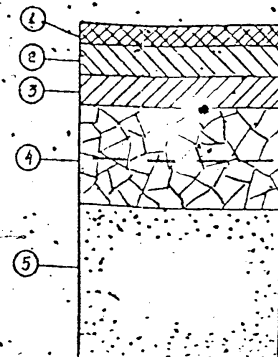
КОНСТРУКЦИИ ТИПА Б-2
